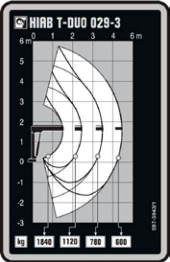
Load diagram HIAB T-DUO 029-3
