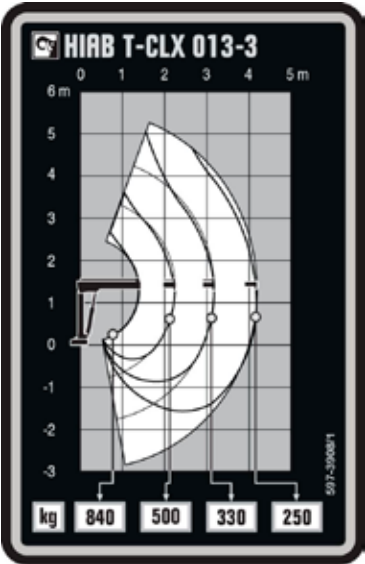
Load diagram HIAB T-CLX 013-3
